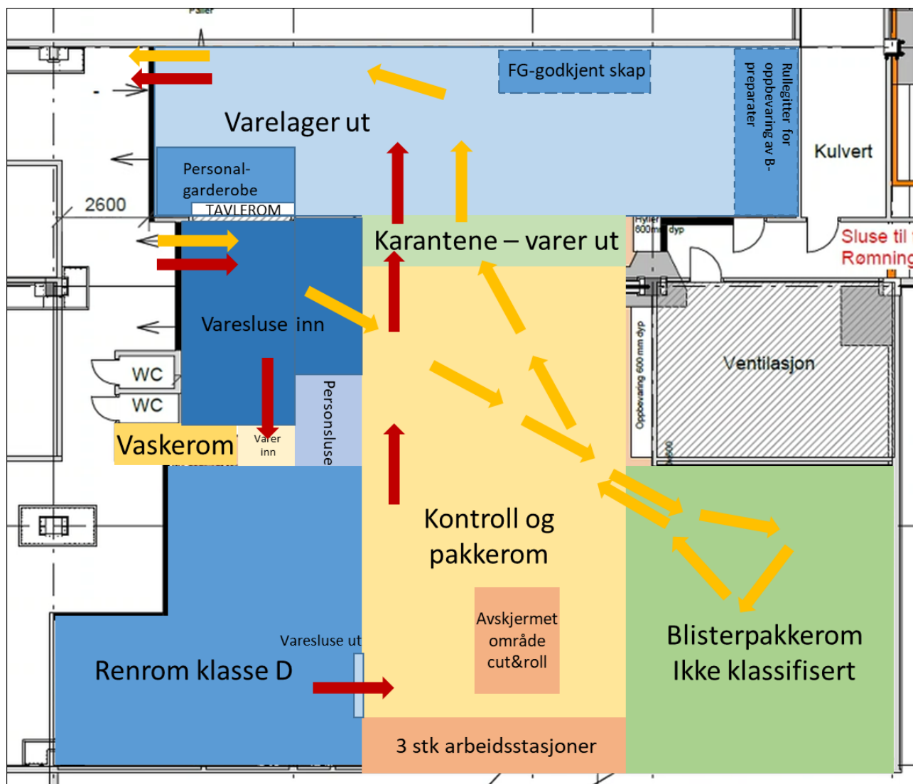
Figur 1 Grov skisse for utforming av pakkeanlegg. Raud pil viser vareflyt for ompakking av lause tablettar/kapslar, medan gul pil viser vareflyt for ompakking av tablettar/kapslar på blisterform.
